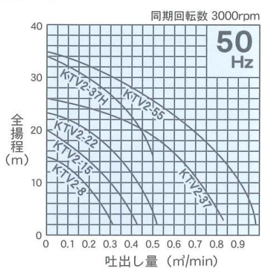
■性能曲線
